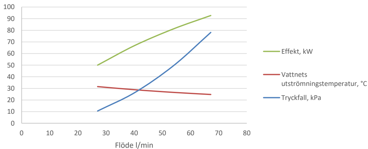
LK L, Tank 40°C, Vatten in 5°C
