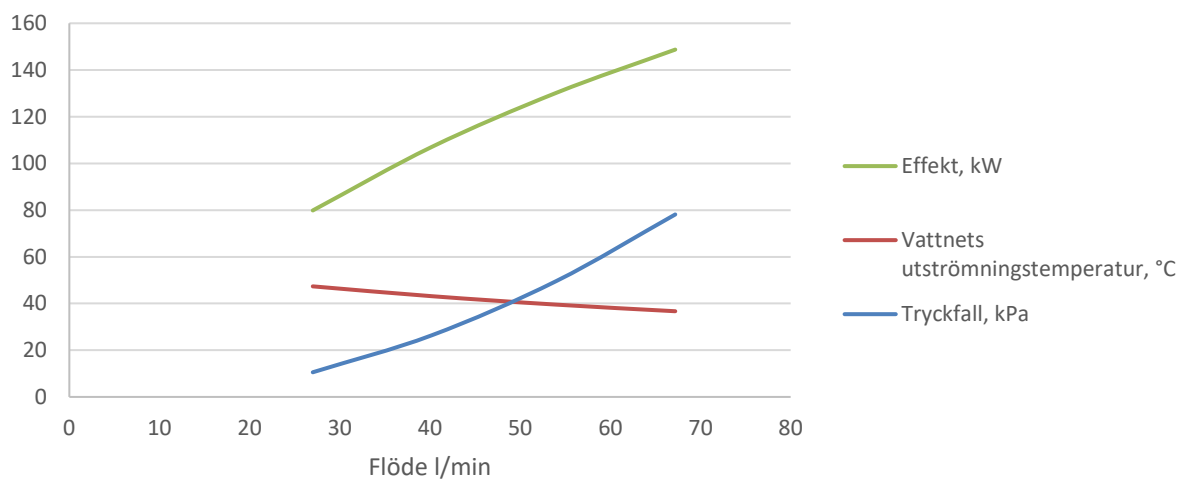
LK L, Tank 60°C, Vatten in 5°C
