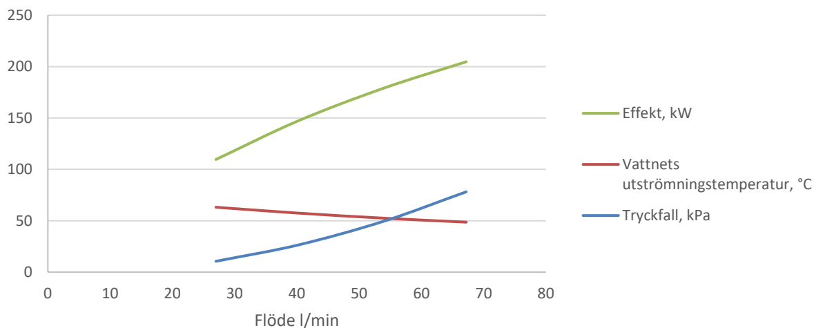
LK L, Tank 80°C, Vatten in 5°C
